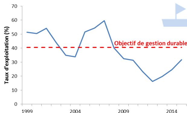
Figure 5. Evolution du taux d'exploitation du stock de merlan de mer Celtique (Source : CIEM, 2016)
