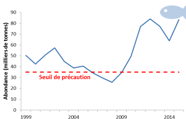
Figure 4. Evolution de l'abondance de reproducteurs du stock de merlan de mer Celtique (Source : CIEM, 2016)
